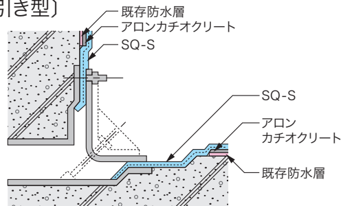
改修用二重ドレン(既存：保護アスファルト防水)
