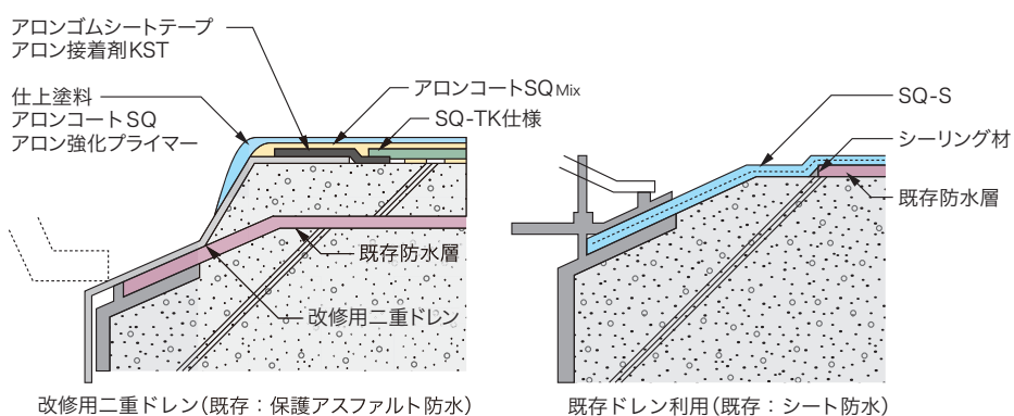
改修用二重ドレン(既存：保護アスファルト防水)
