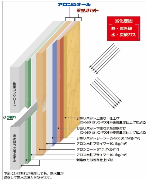
【アロンウオール ジョリパット工法の工程図】
